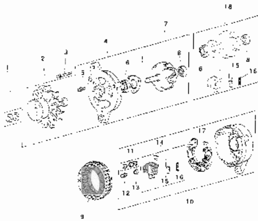
FIG. 118 ALTERNATOR
