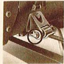
33. Brida de ballesta en la izquierda.
