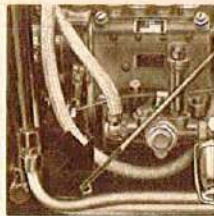
2. Comprobar nivel de aceite en el motor.
