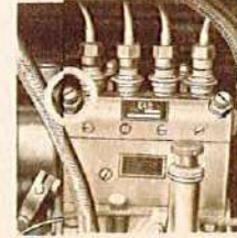
37. Cambio de aceite en la bomba de inyección.
