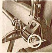
36. Brida de ballesta en la derecha.
