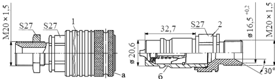
1 – полумуфта охватывающая НР10-1-Х0044; 2 – полумуфта охватываемая НР10-2-Х0041; а – втулка; б – канавка
