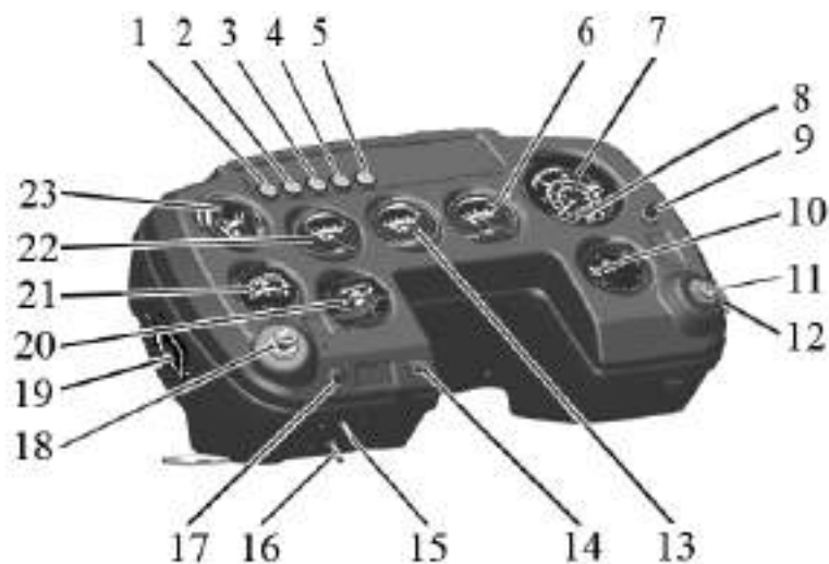
Рисунок 7 – Панель приборов
