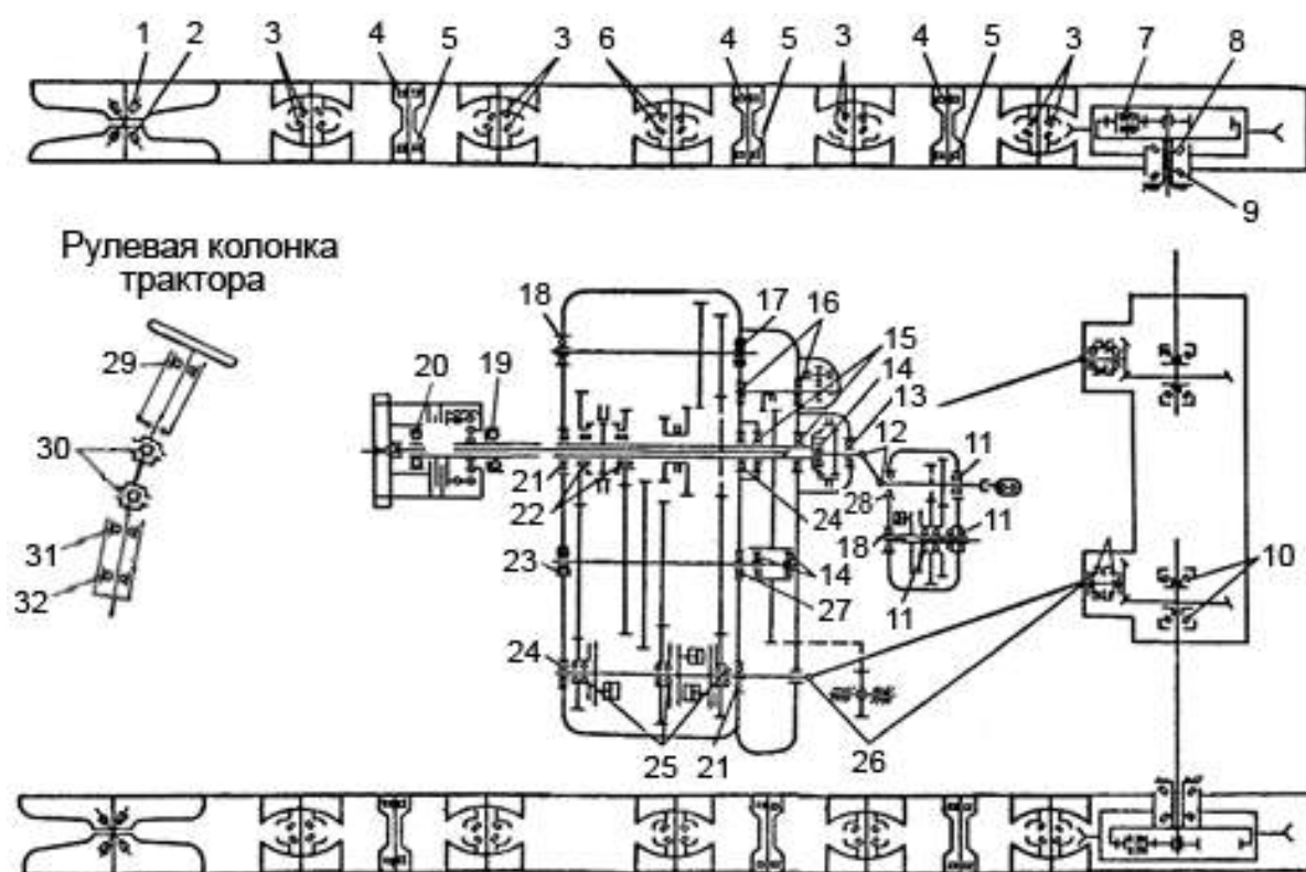
Рисунок 83 – Схема расположения подшипников на тракторе
