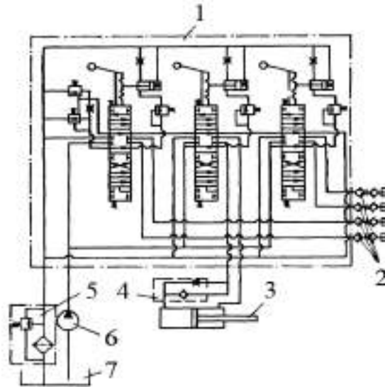
1 – распределитель; 2 – муфты соединительные; 3 – гидроцилиндр; 4 – клапан замедлительный; 5 – фильтр магистральный; 6 – насос; 7 – бак масляный
