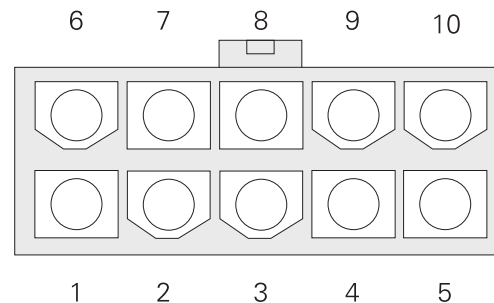
Vista de Frente Conector - Distribución de Terminales
