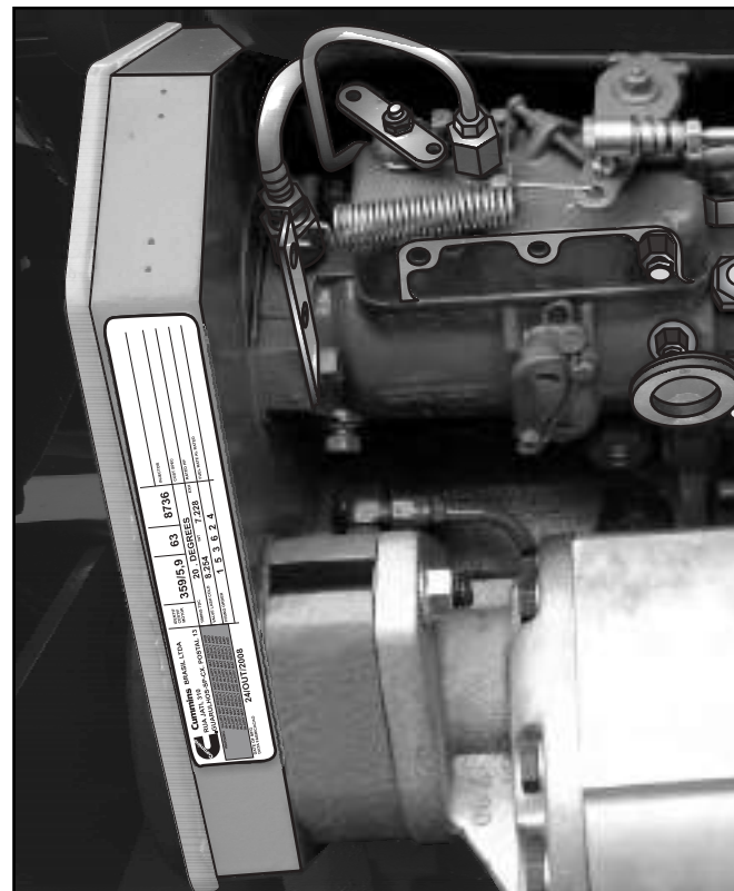
Ubicación de la Placa identificativa del motor Cummins
