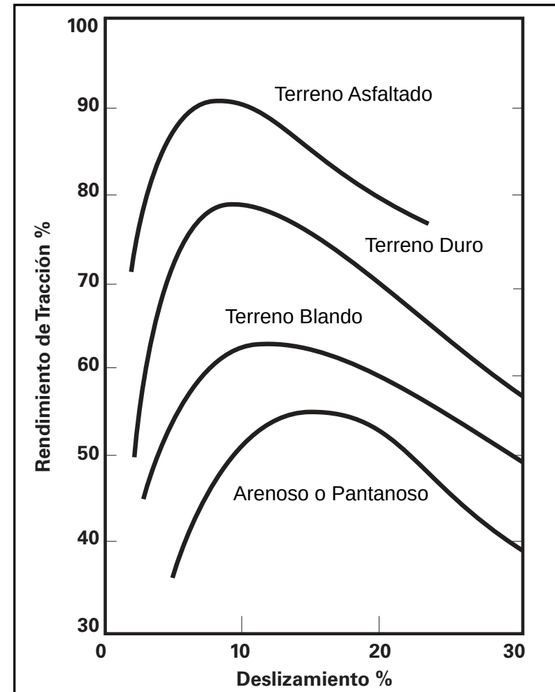
Rendimiento de Tracción en Tractores Agrícolas
