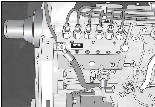
Bomba Inyectora Lineal
