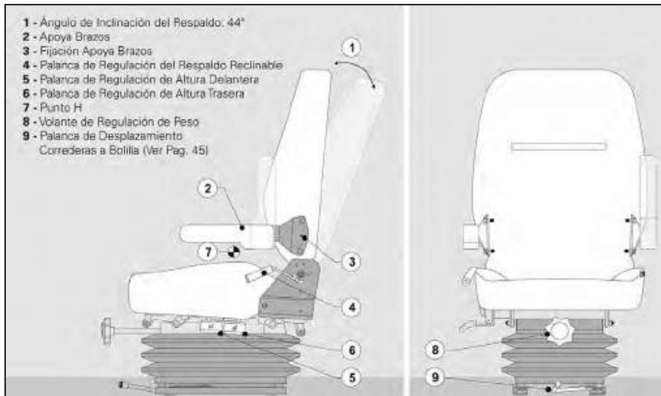
Asiento del Operador
